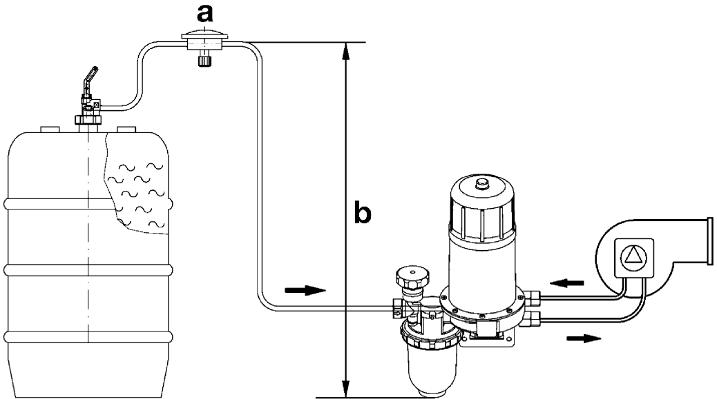
Bild 4: Einbaubeispiel eines FloCo-TOP unterhalb des Tankspiegels.
