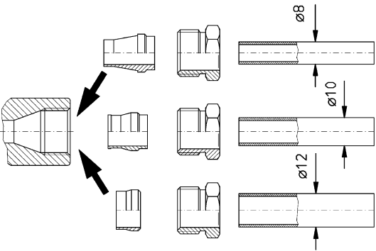
Bild 2: AFRISO Universal-Rohrverschraubung
